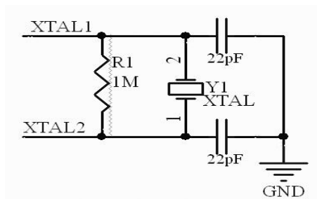
外部晶振参考电路
