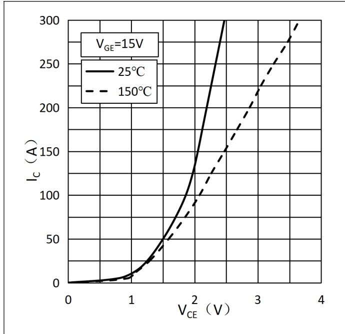
I_c=f(V_{CE}), V_{GE}=15V Fig.1 Typ. Output Characteristics-Inverter 图 1 输出特性-逆变器
