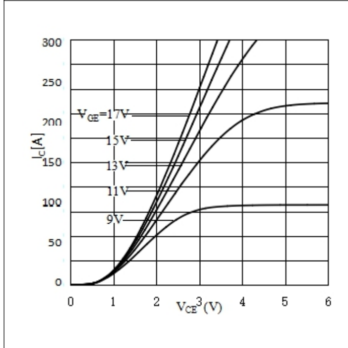
I_c=f(V_{CE}), T_{vj}=150^\circ C Fig.3 Typ. Output Characteristics-Inverter 图 3 输出特性-逆变器
