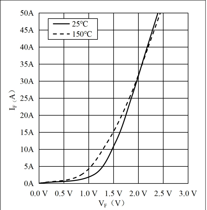
图 10 二极管正向偏压特性-整流器
