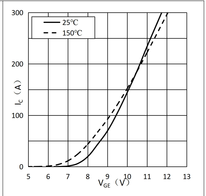
I_c=f(V_{GE}), V_{CE}=20V Fig.2 Typ. Transfer Characteristics-Inverter 图 2 传输特性-逆变器
