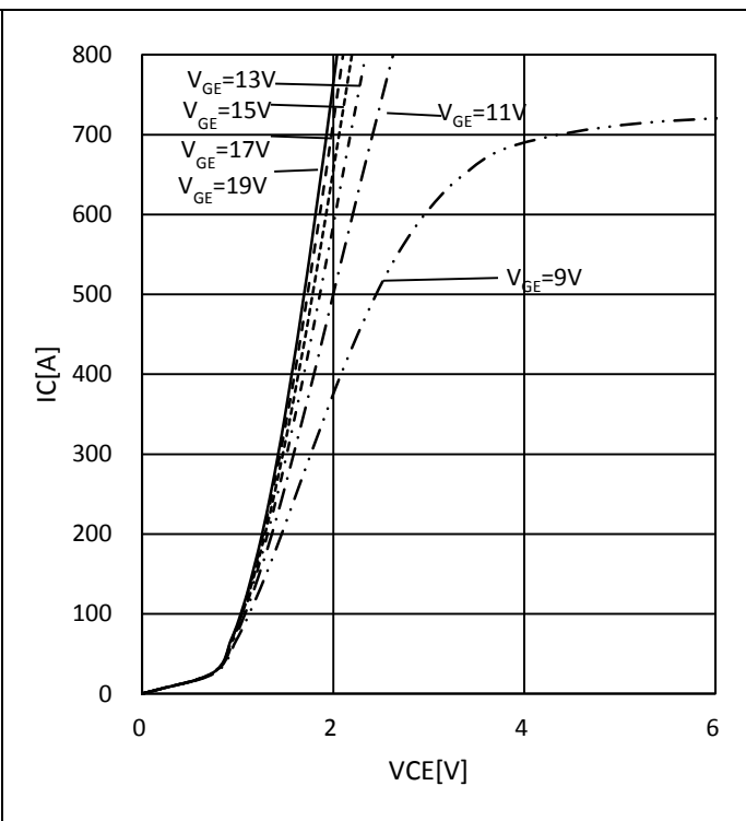
T_{vj} = 150^\circ C Fig.2: Output characteristics 图 2: 输出特性
