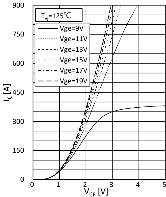
Fig.3 Output Characteristics 图 3 输出特性
