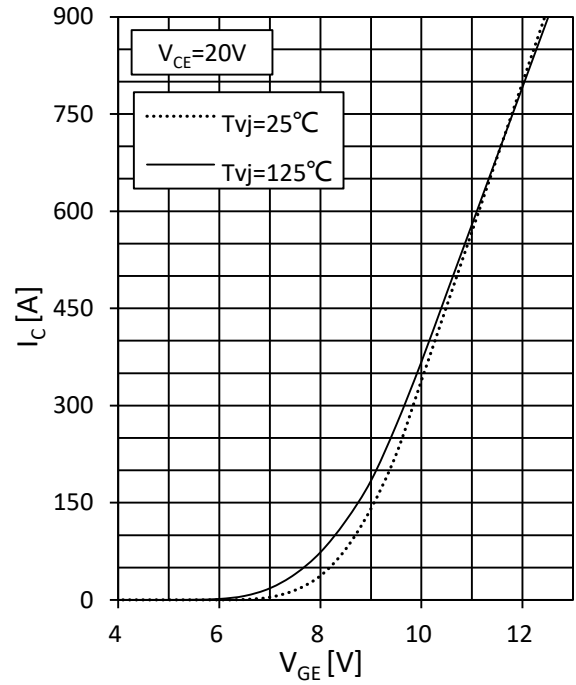
Fig.2 Transfer Characteristics 图 2 传输特性
