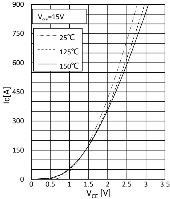
Fig.1 Output Characteristics 图 1 输出特性
