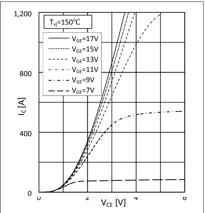
Fig.2: Output characteristics 图 2: 输出特性
