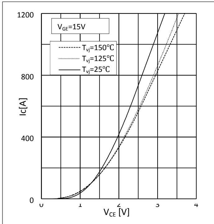
Fig.1: Output Characteristics 图 1: 输出特性
