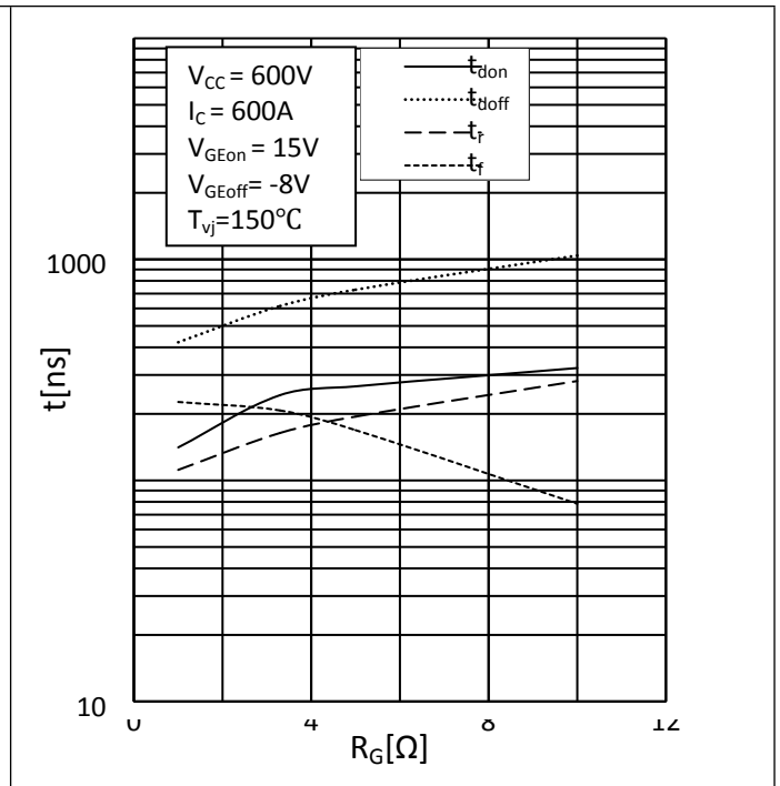
Fig.6: Switching Times vs. Gate Resistor 图 6: 开关时间与门极电阻关系
